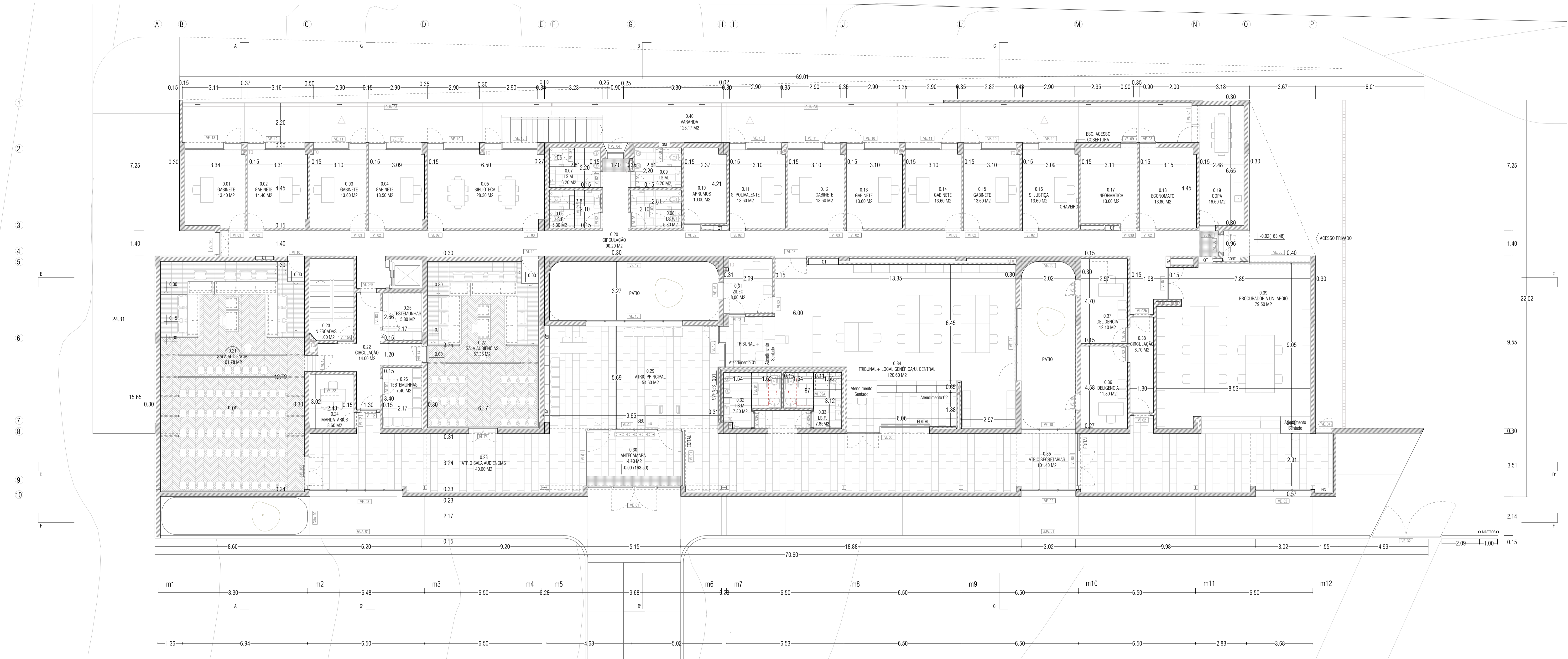
PLANTA PISO 0 1:100
